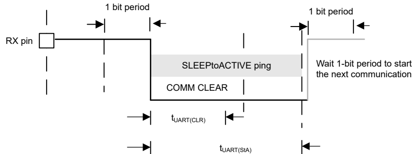
図 8-19. UART COMM CLEAR
