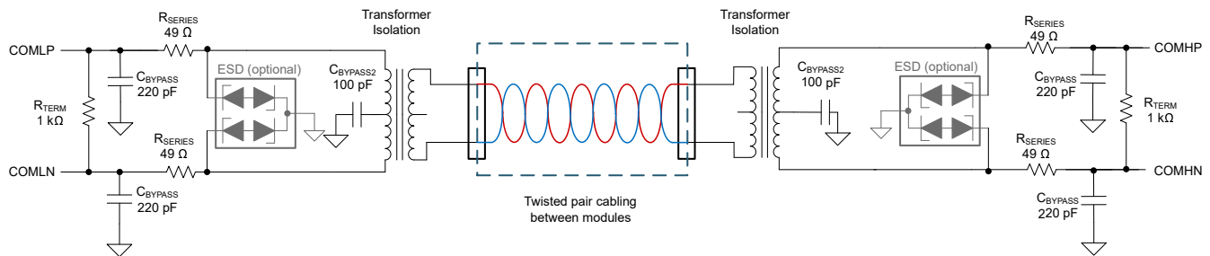
图 9-9. Transformer Isolation
