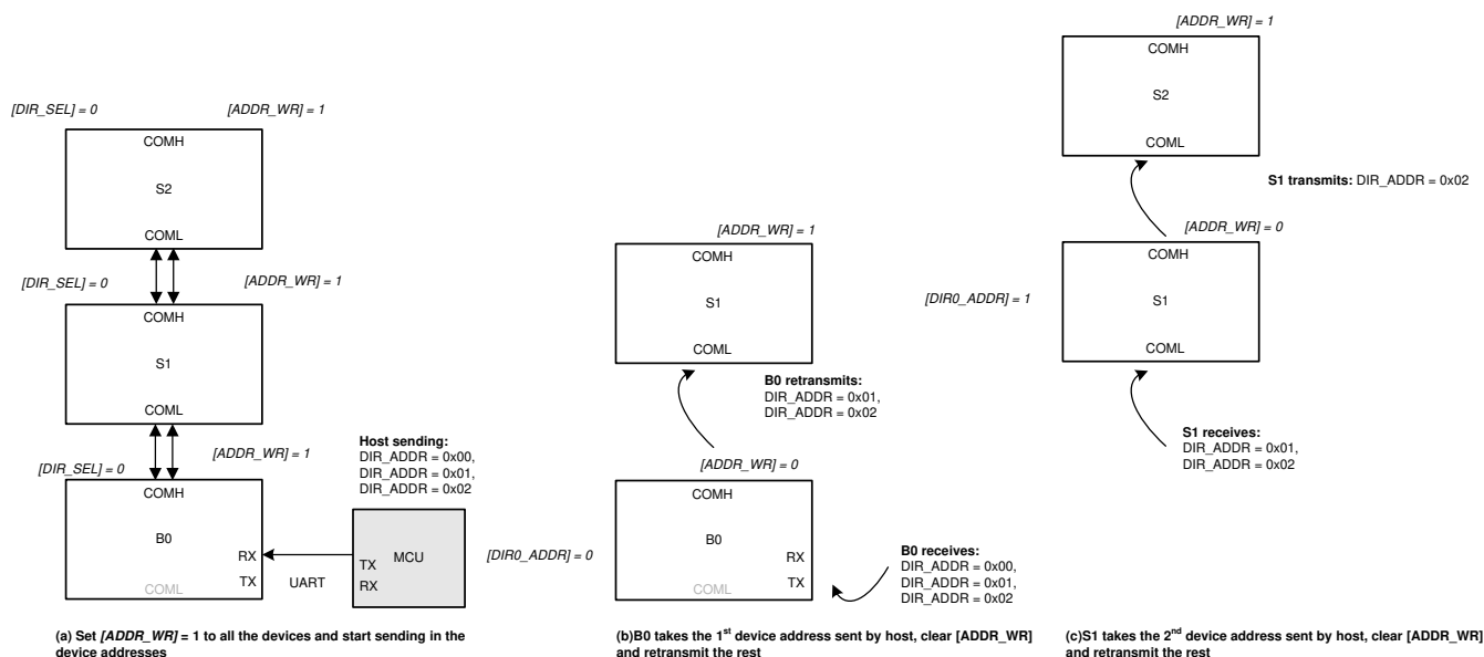
图 8-36. Auto-Addressing
