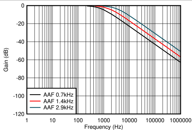
7-6. AUX ADC Filter
