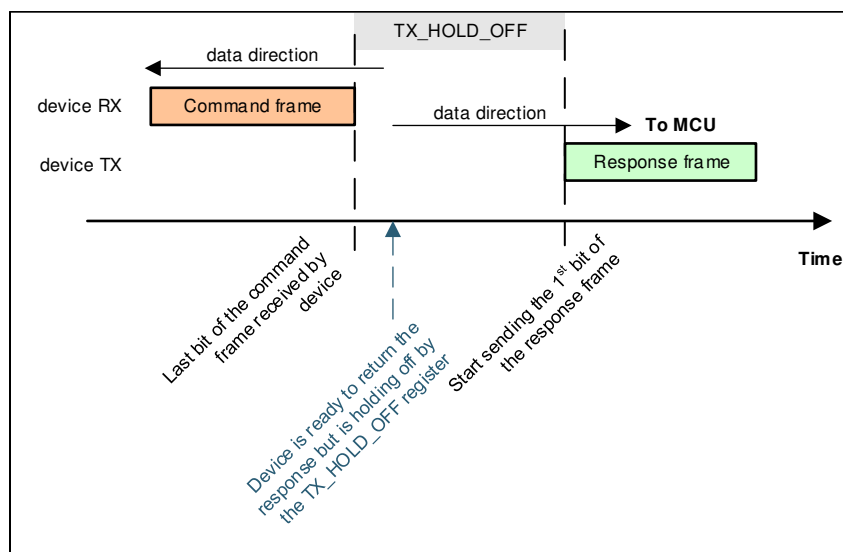
图 9-25. UART TX_HOLD_OFF
