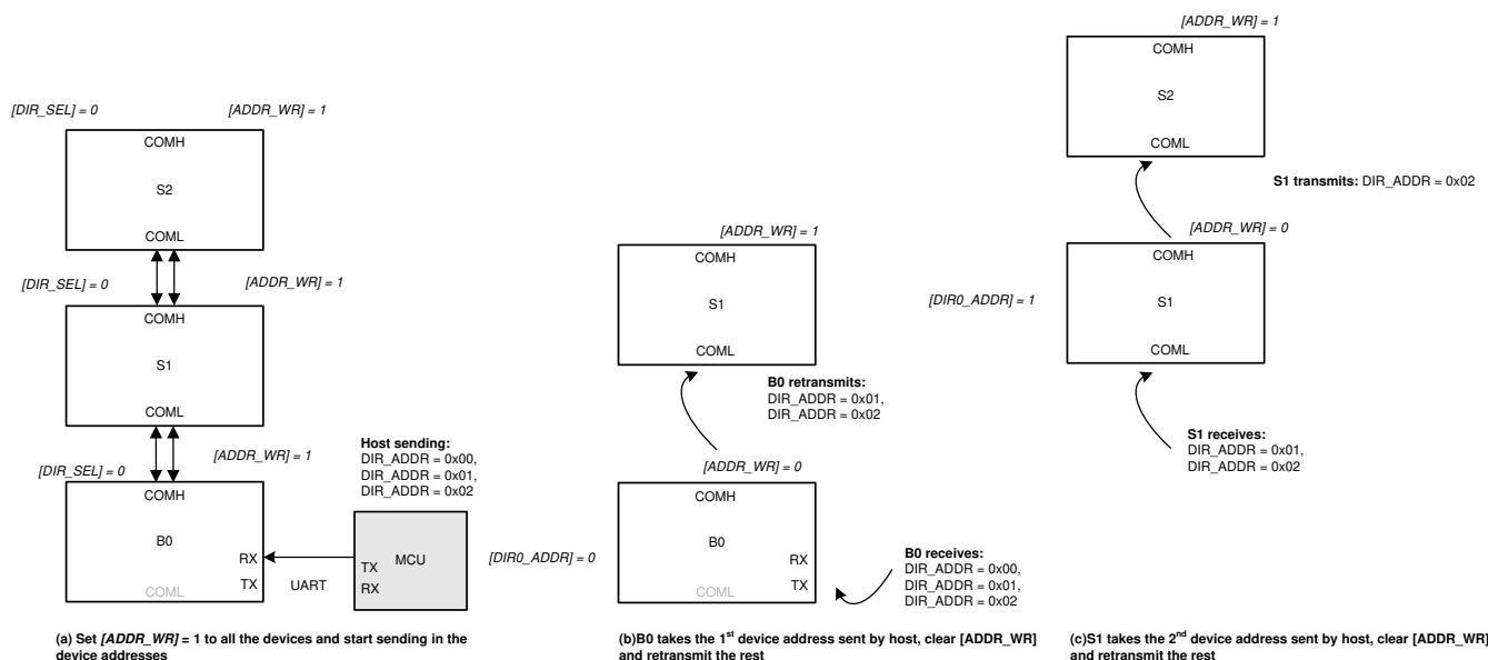
图 9-36. Auto-Addressing
