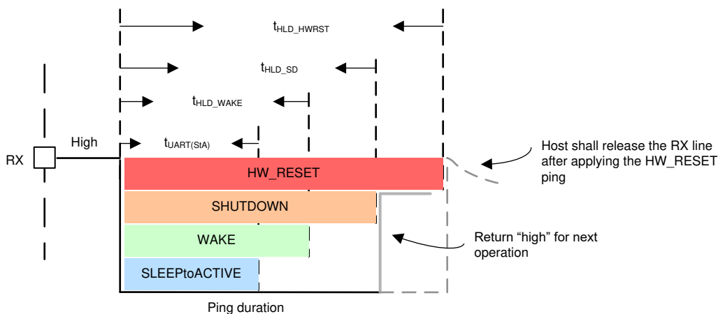
図 9-62. Communication Pings
