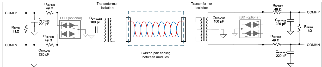
图 10-9. Transformer Isolation
