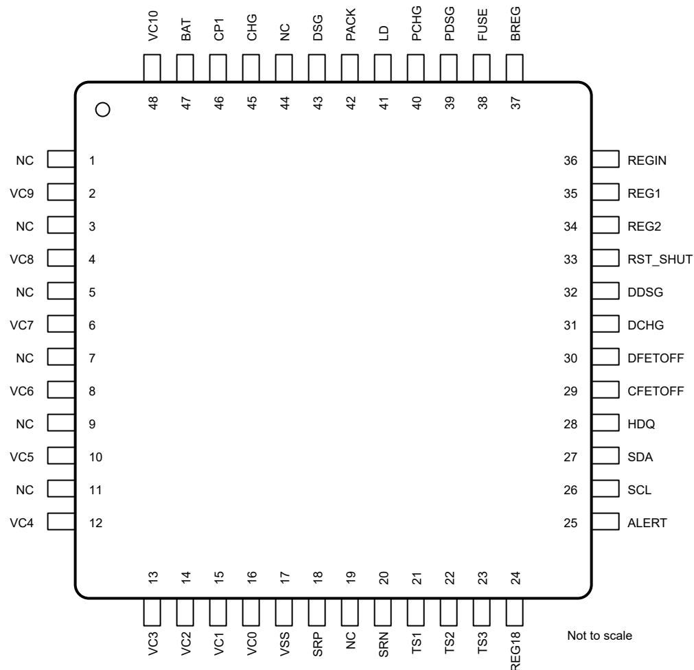
図 6-1. Pinout (top)
