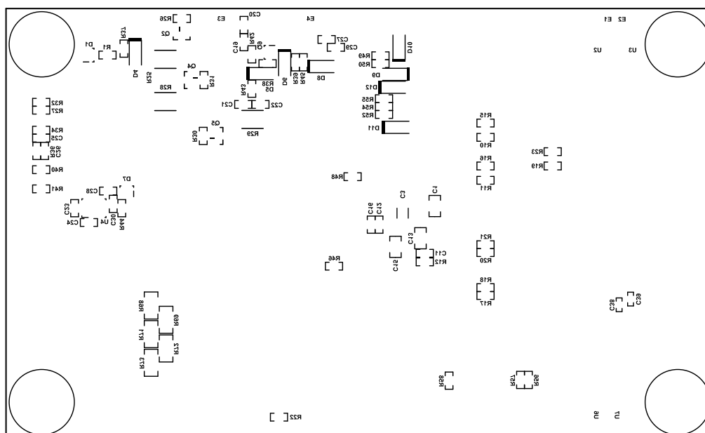
10-6. BQ76922EVM Bottom Layer
