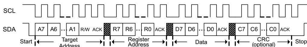
図 7-1. I 2 C Write
