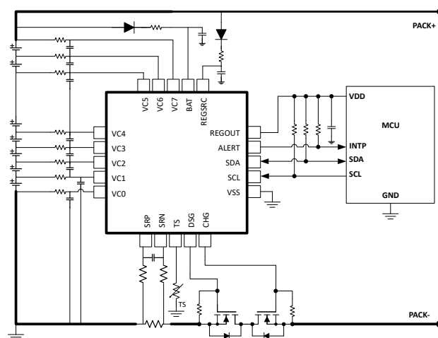
概略回路図
