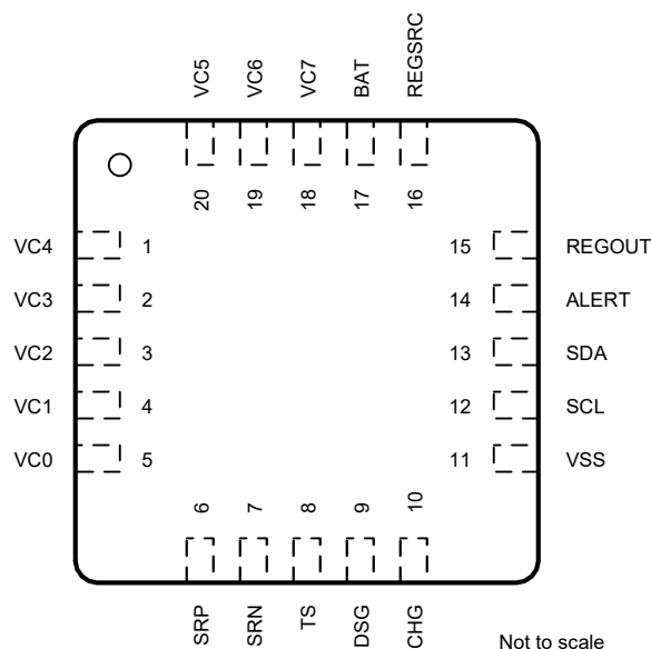
図 5-1. BQ76907 Pinout
