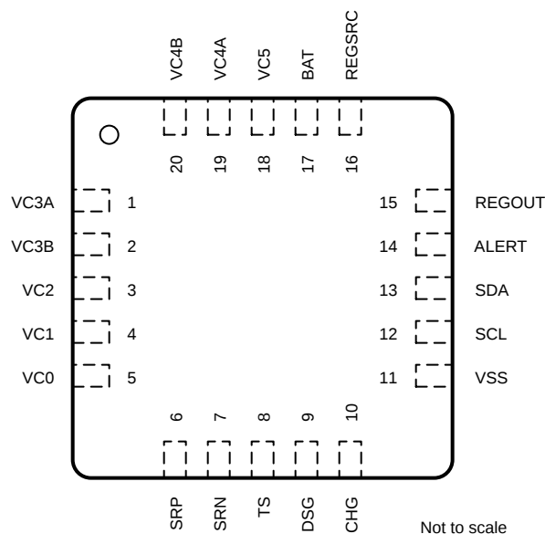
図 5-1. BQ76905 Pinout
