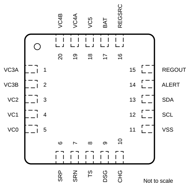
図 5-1. BQ76905 Pinout
