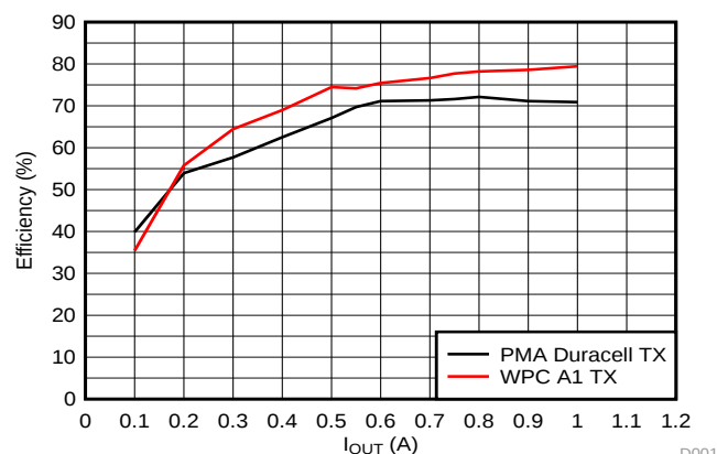
5V出力のデュアル・モード効率
