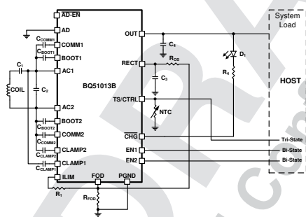
簡略回路図
