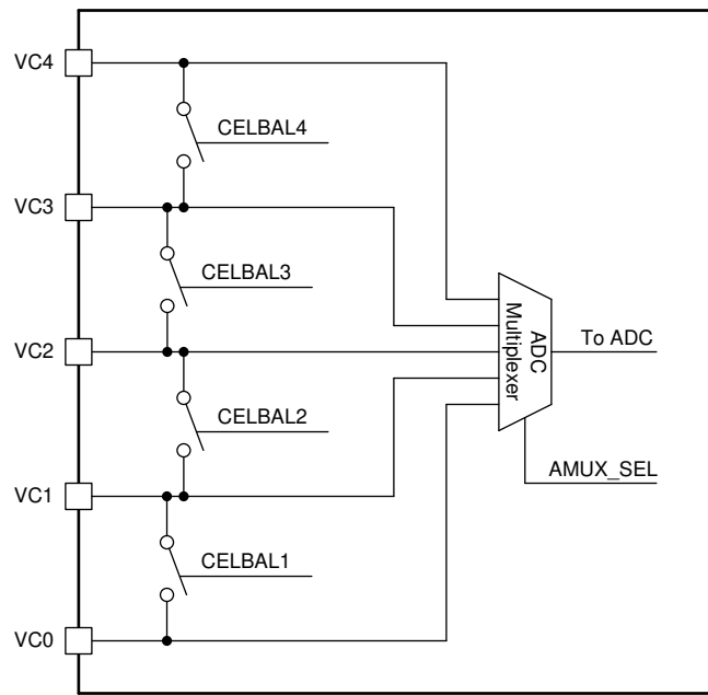
図 5-2. VCx Pins
