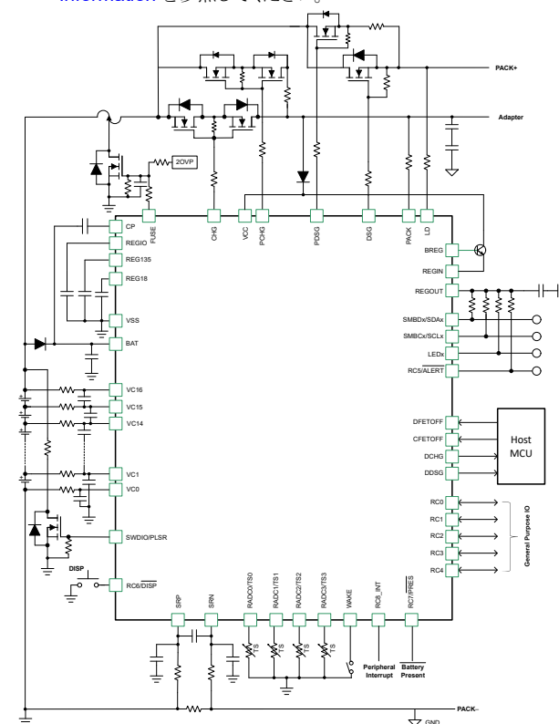
概略回路図
