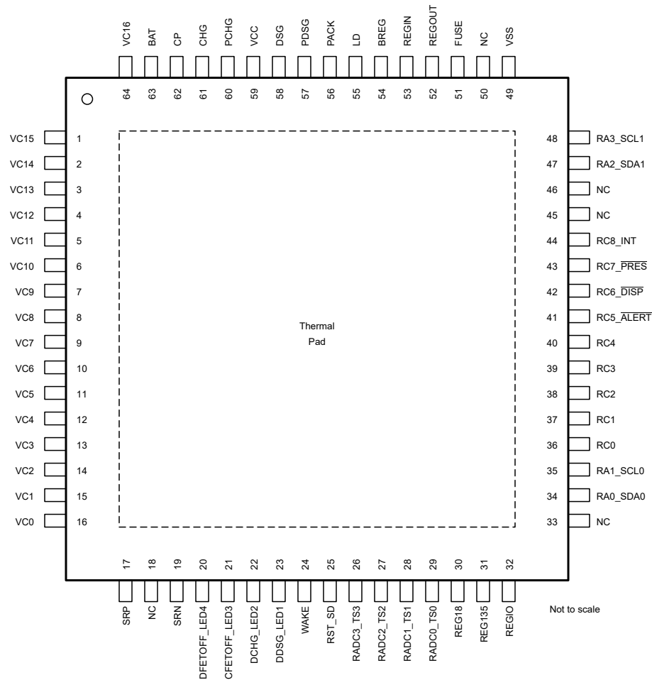
図 4-1. Pin Diagram
