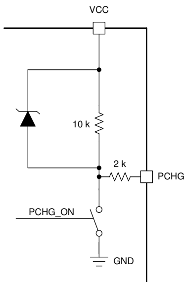
図 5-7. PCHG Pin
