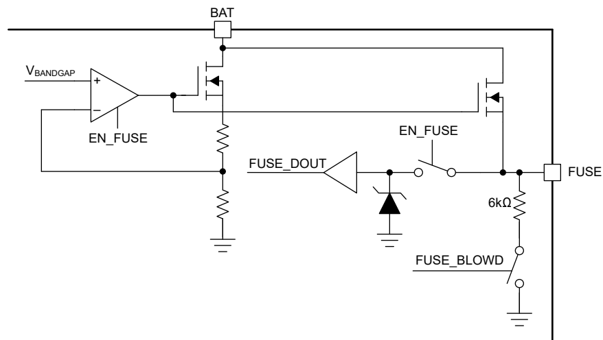
図 5-4. Fuse Pin
