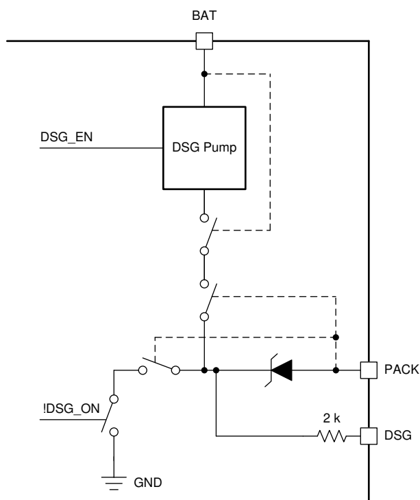
図 5-6. DSG Pin
