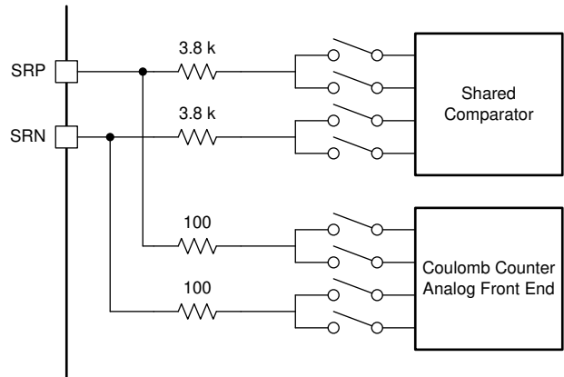
図 5-1. SRx Pins
