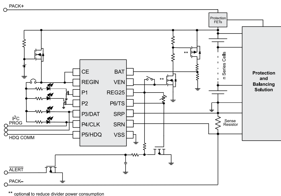
簡略回路図
