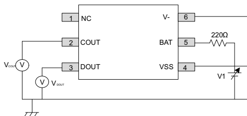
図 7-3. Test Circuit 1
