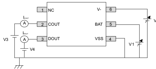
図 7-6. Test Circuit 4
