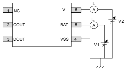
図 7-5. Test Circuit 3
