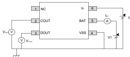
図 7-4. Test Circuit 2
