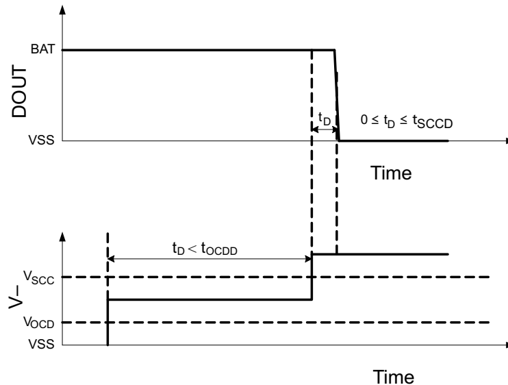
図 8-1. Delay Circuit
