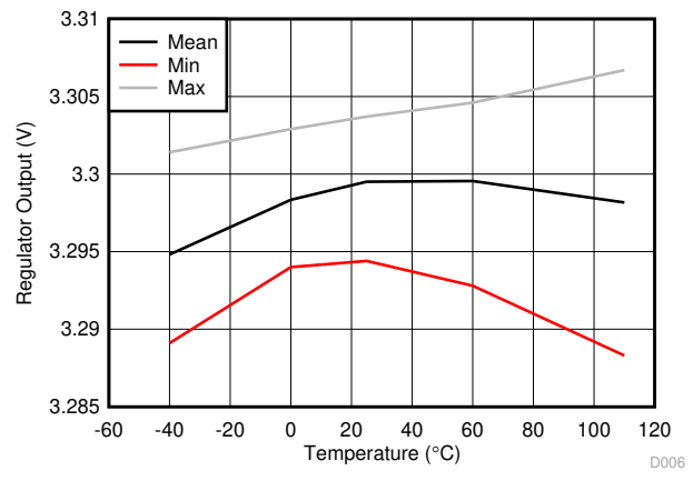
図 6-6. 負荷なしのレギュレータ出力
