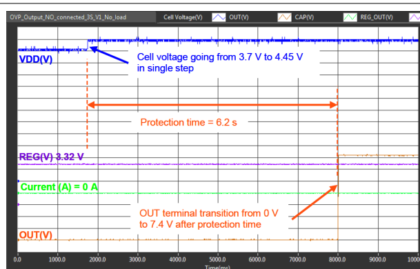
図 8-4. 過電圧保護
