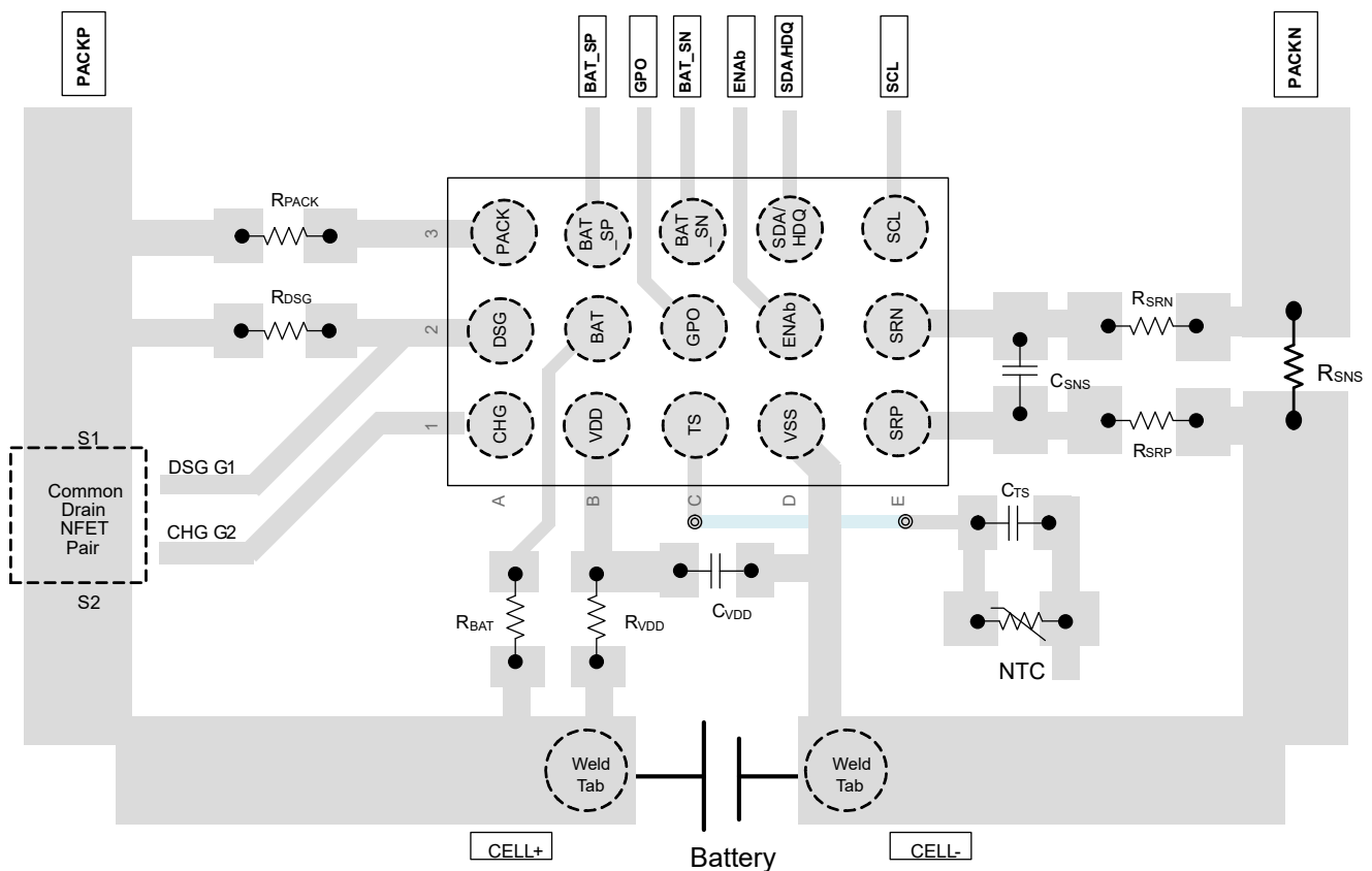
図 9-1. BQ27Z758 の主要トレース基板レイアウト
