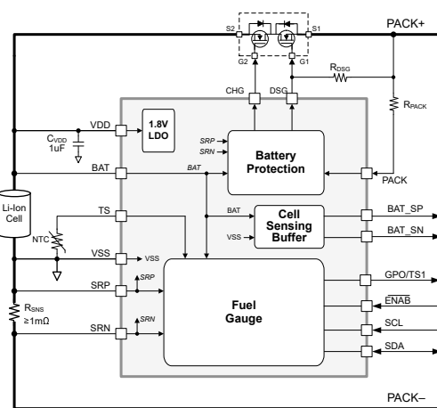
BQ27Z758 の概略回路図
