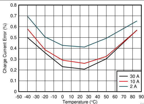
図 5-3. 充電電流誤差と温度および充電器電流との関係 (1mΩ センス抵抗使用、キャリブレーションなし)
