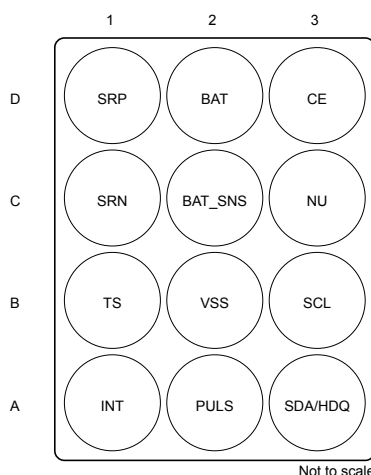
図 6-1. Pin Diagram
