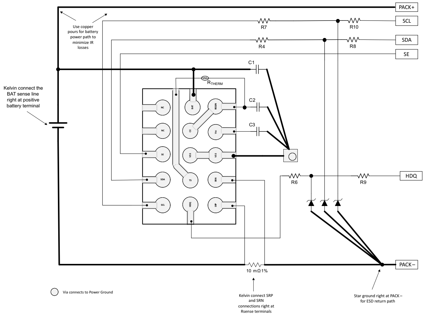
✶ 14. Layout Example
