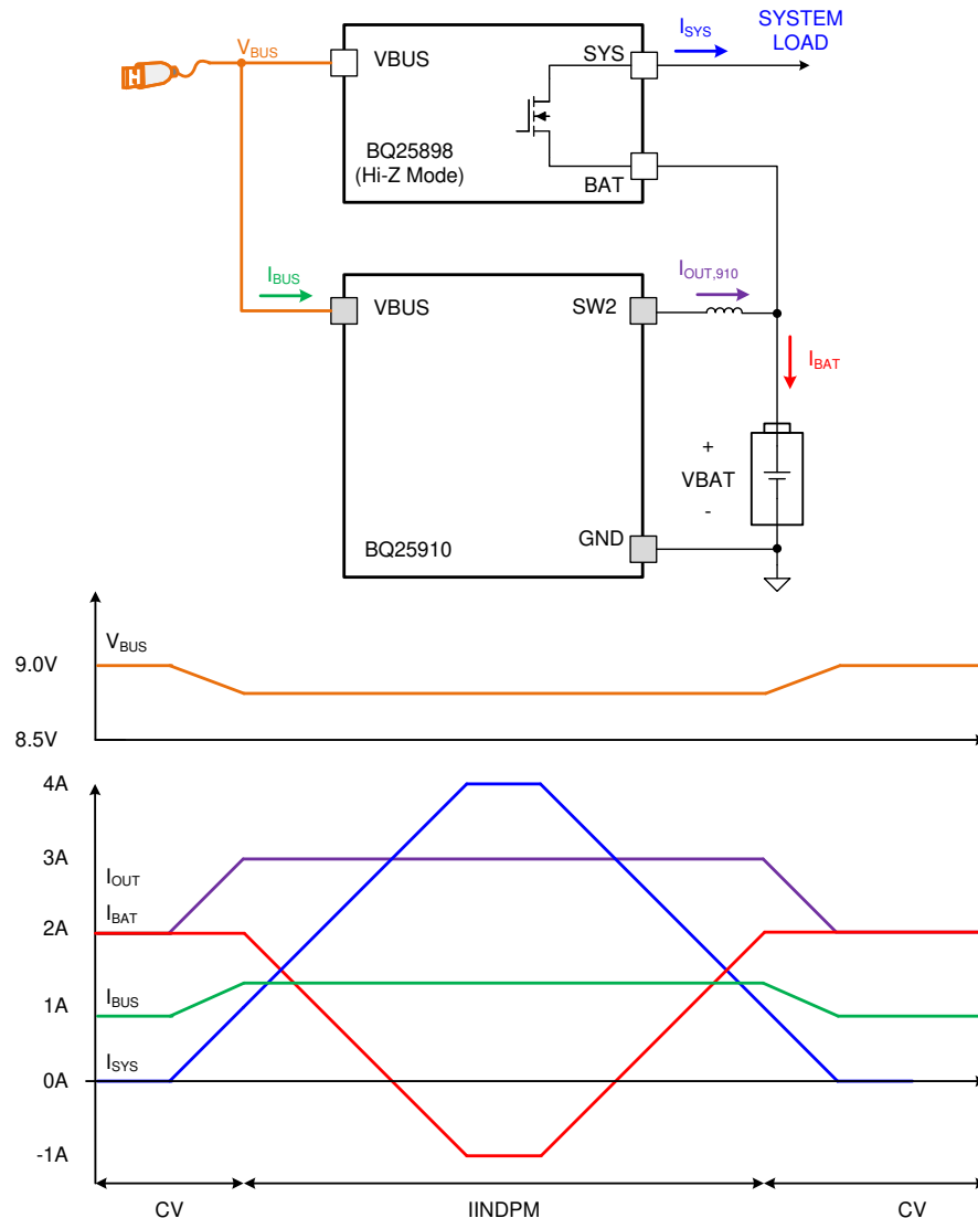
图 20. DPM Response
