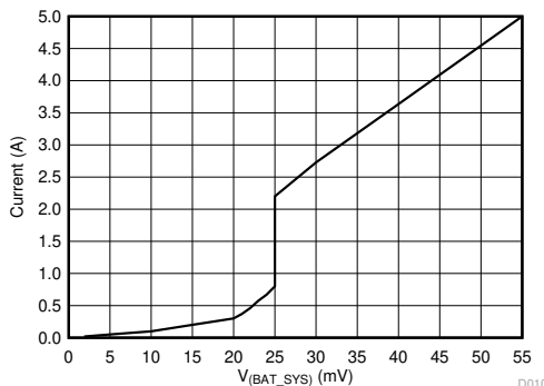
図 9-4. BATFET V-I Curve
