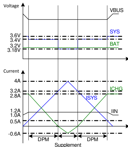
図 9-3. DPM Response
