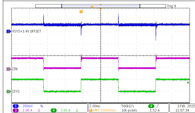
10-4. Charge Enable
