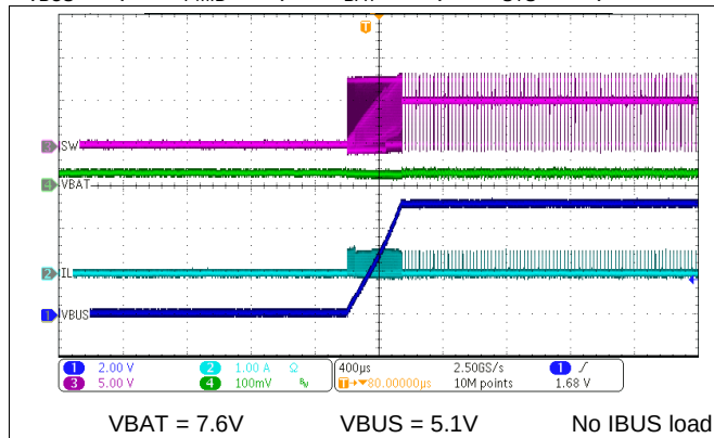
图 82. Buck Mode (OTG) Startup
