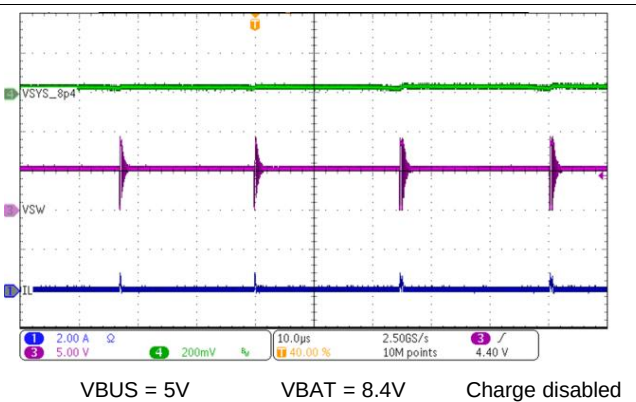
图 87. Boost Mode PFM Switching
