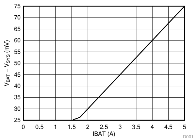
FIG 21. BATFET I-V Curve
