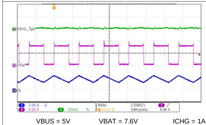
图 86. Boost Mode PWM Switching
