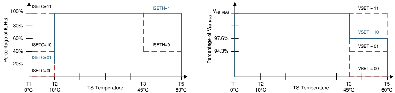
図 7-4. TS Charging Values
