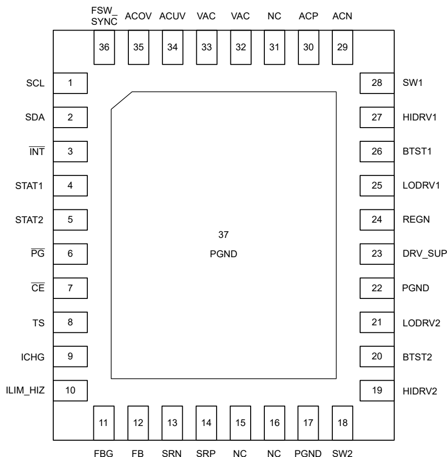
図 5-1. BQ25856-Q1, RRV Package 36-Pin VQFN Top View
