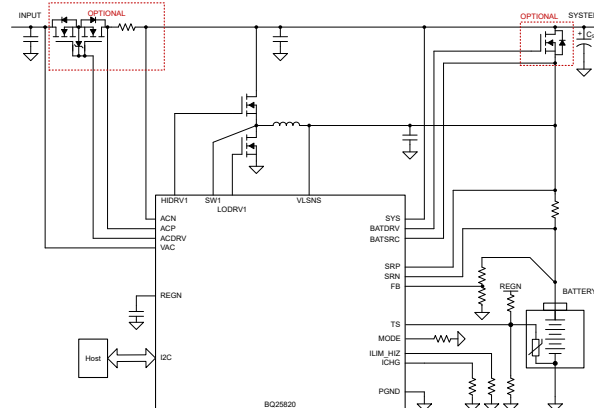
BQ25820 の概略回路図
