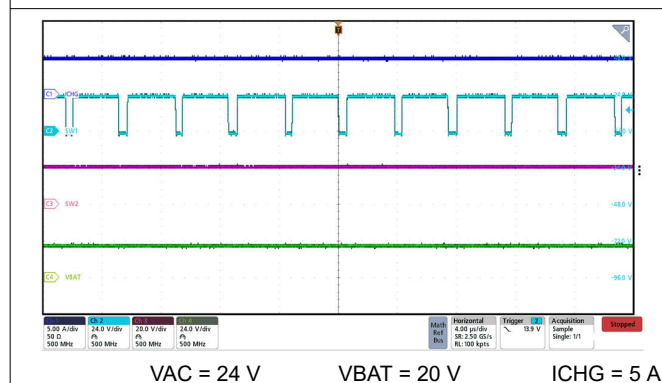
図 8-7. Buck Switching Waveform
