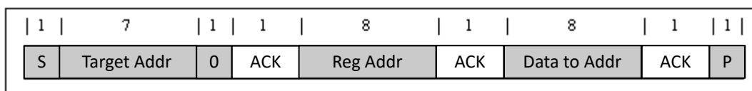
図 7-11. Single Write
