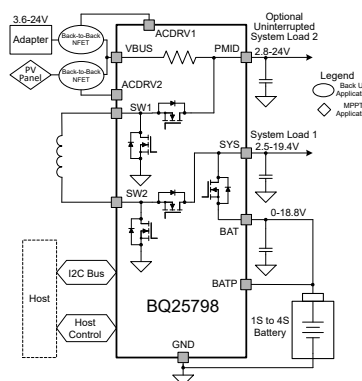
簡略回路図
