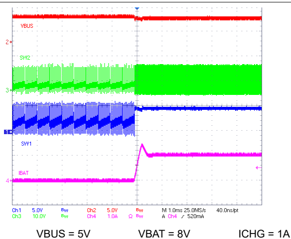
10-6. Charge Enable
