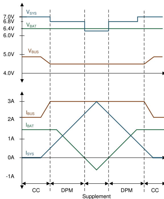
图 9-9. DPM Response
