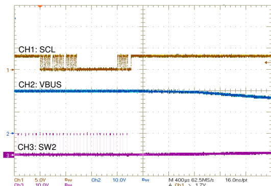
図 10-16. OTG Power Off
