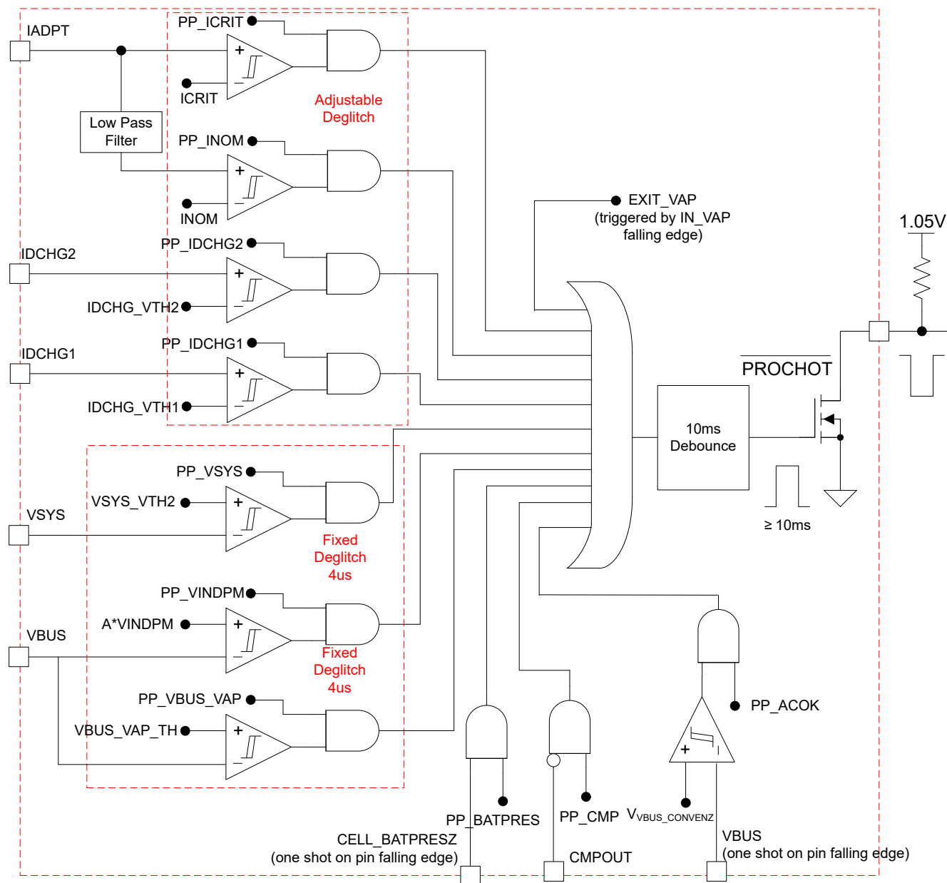
图 9-4. \overline{\text{PROCHOT}} Profile
