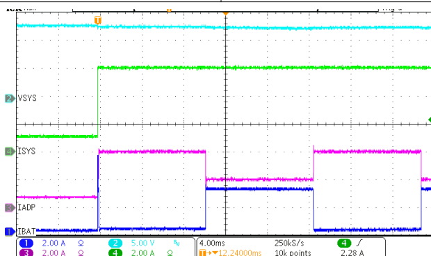
図 10-17. OTG Load Transient
