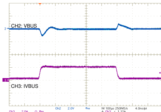
図 10-17. OTG Load Transient
