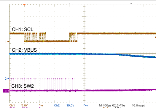
図 9-19. OTG Power Off
