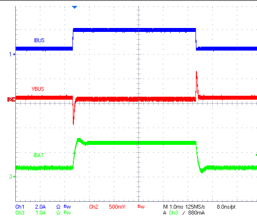
图 9-8. VOTG Load Transient Response
