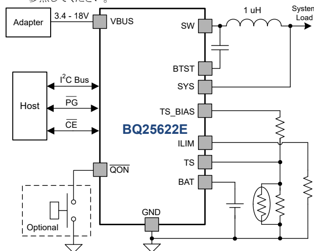
BQ25622E のアプリケーション概略図
