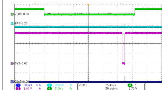
図 9-4. Charge Enable
