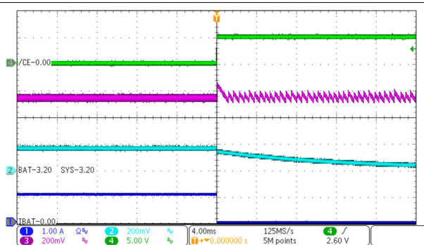
図 9-3. Power-Down
