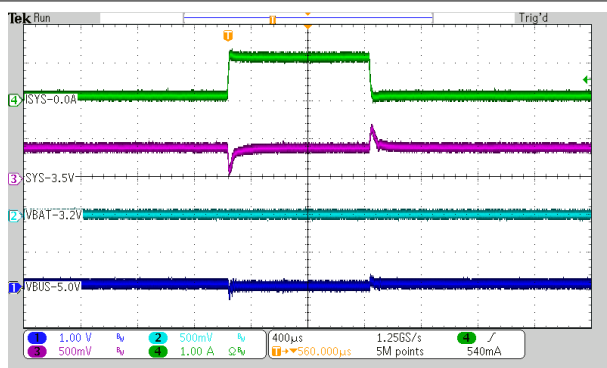
図 9-9. PFM Switching in Buck Mode
