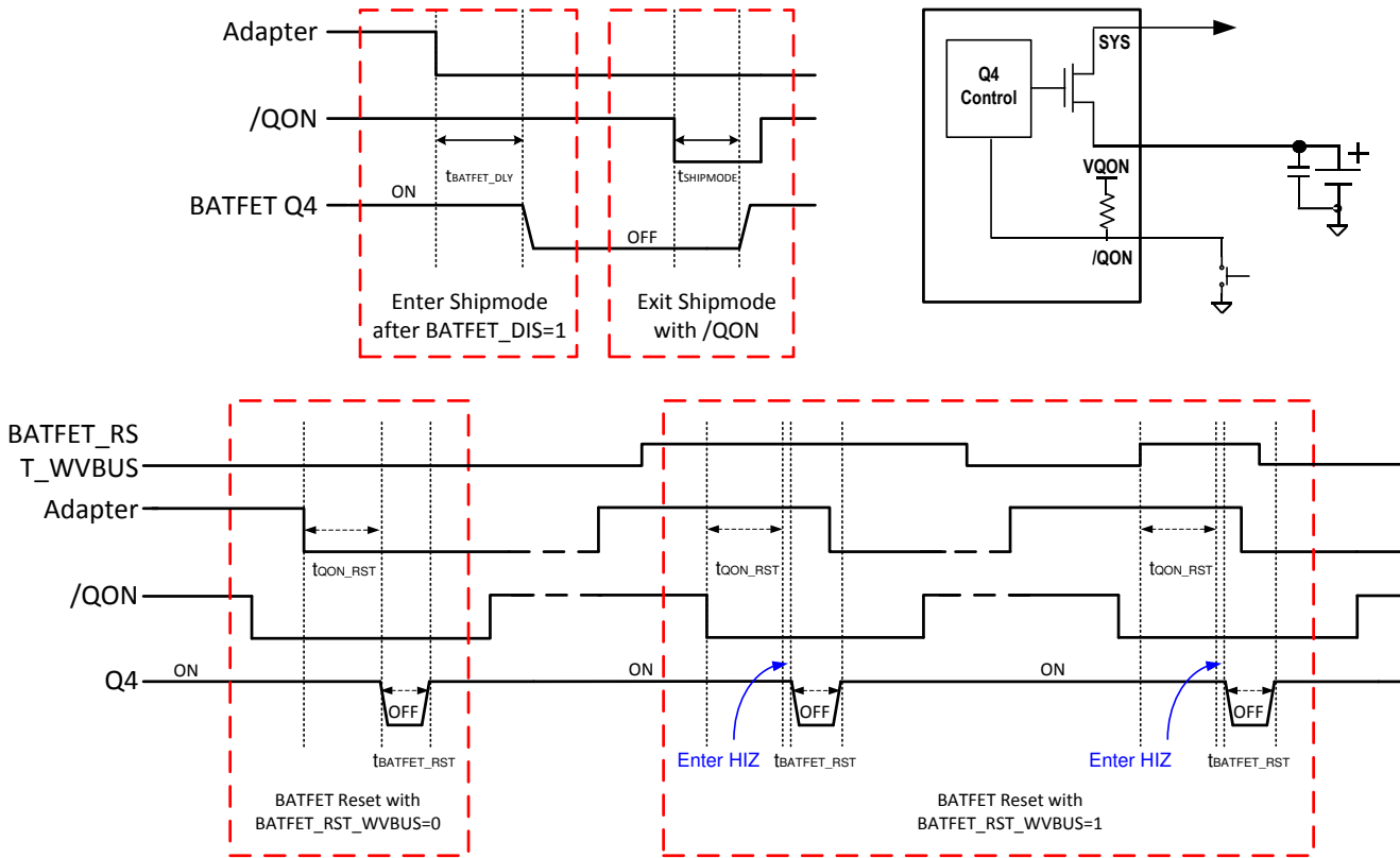
図 7-6. QON Timing
