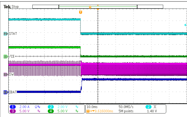
10-9. Charge Enable
