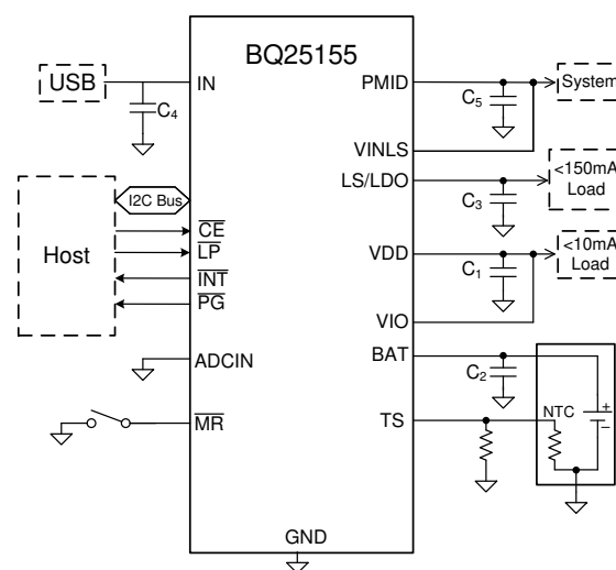
概略回路図
