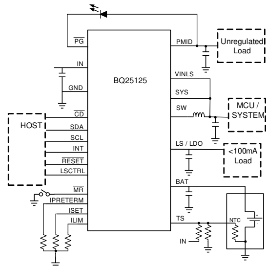
概略回路図
