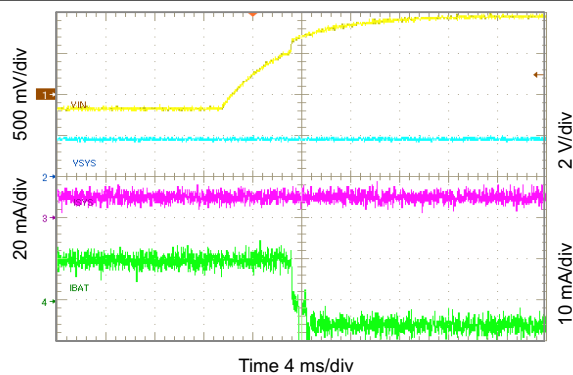
10-7. OVP Fault
