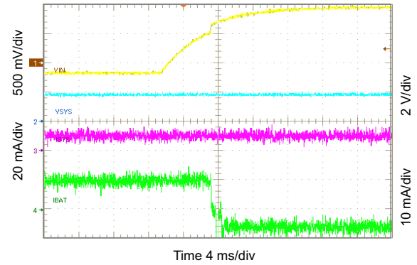
10-9. OVP Fault
