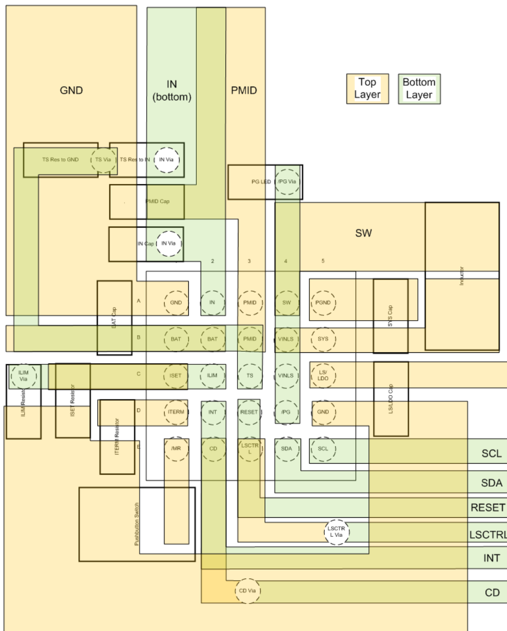
12-1. BQ25121A Layout
