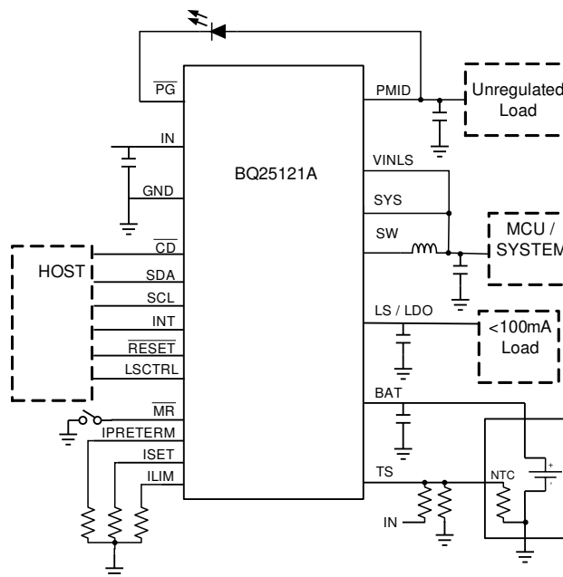
簡略回路図
