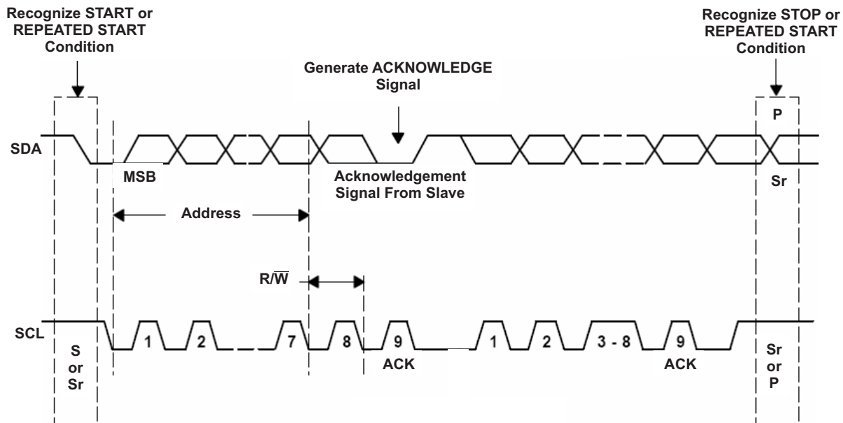
图 22. Bus Protocol
