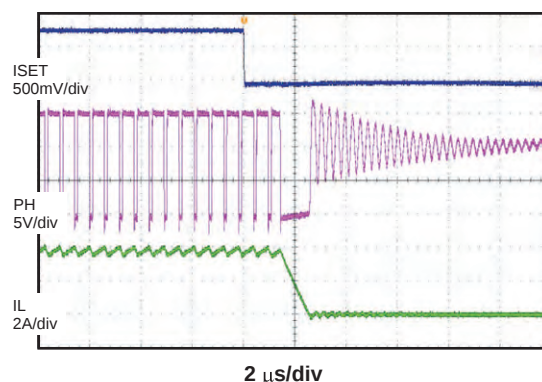
図 6. ISETによる充電ディスエーブル
