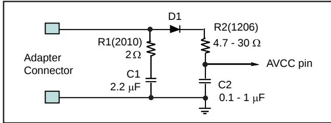
図 22. 入力フィルタ
