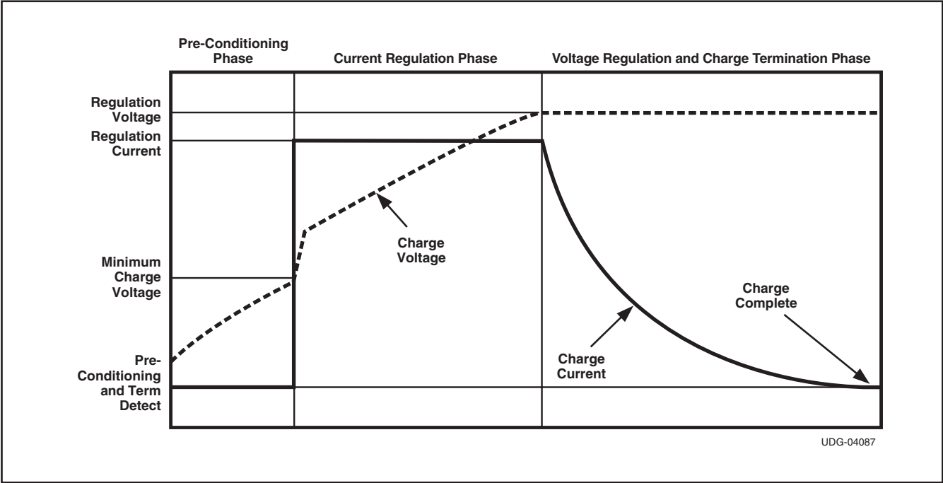
図 1. Charge Profile
