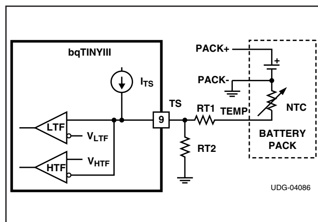
図 15. TS Pin Thresholds
