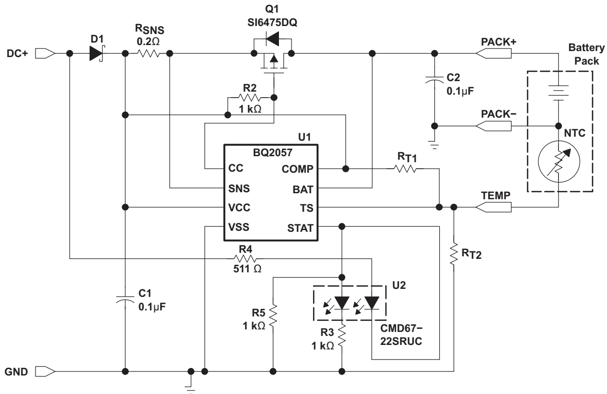
FIG 10-4. 0.5-A Charger Using P-Channel MOSFET
