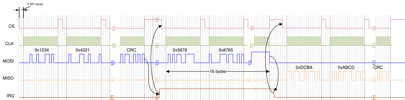
図 7-13. SPI 通信
