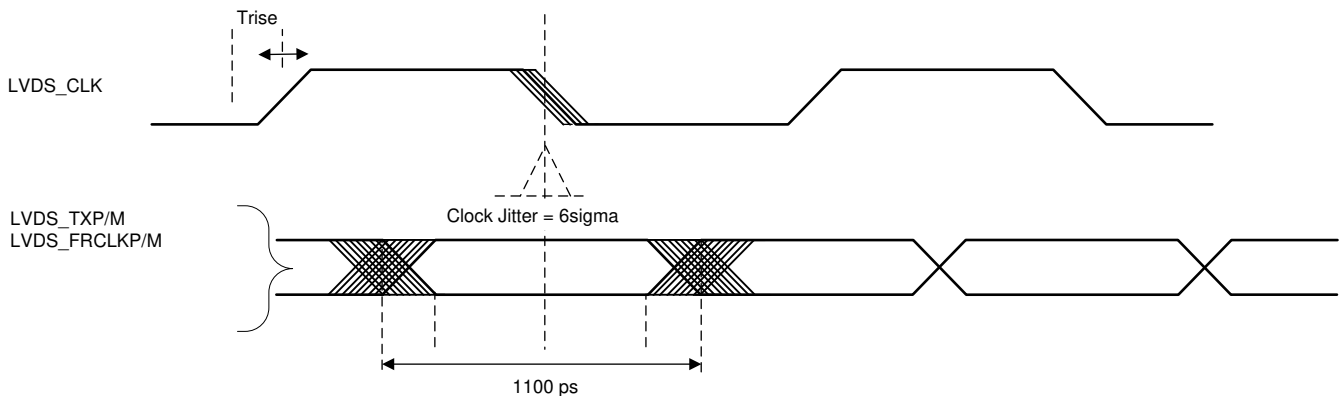
図 7-21. Timing Parameters
