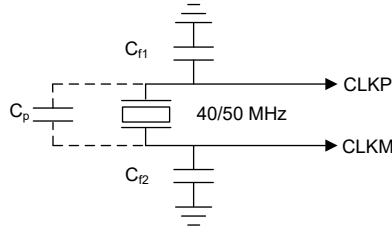
図 7-3. Crystal Implementation
