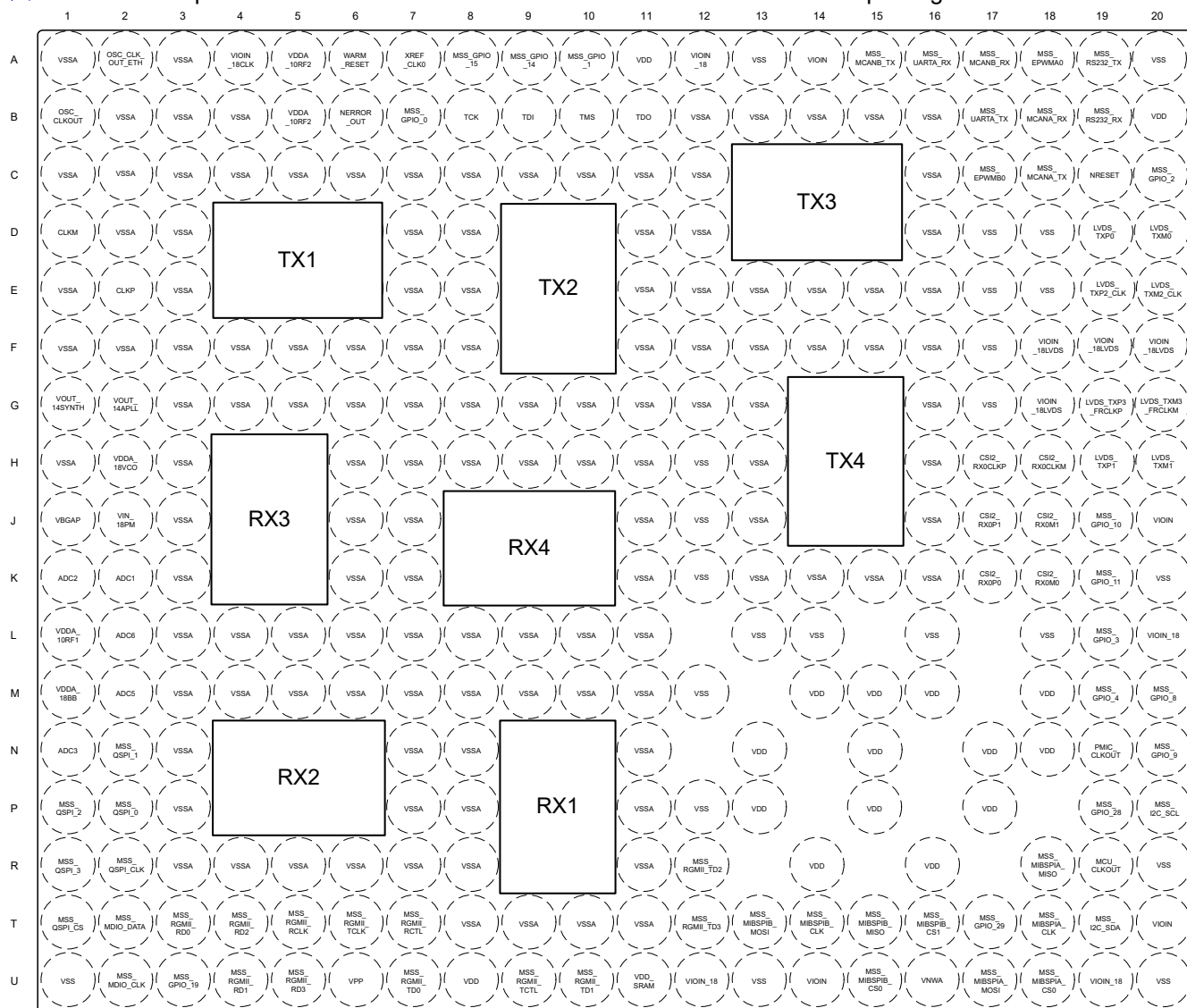
図 6-2. Pin Diagram - AWR2E44P
