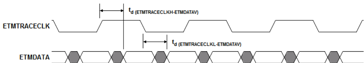
図 7-26. ETMDATA Timing
