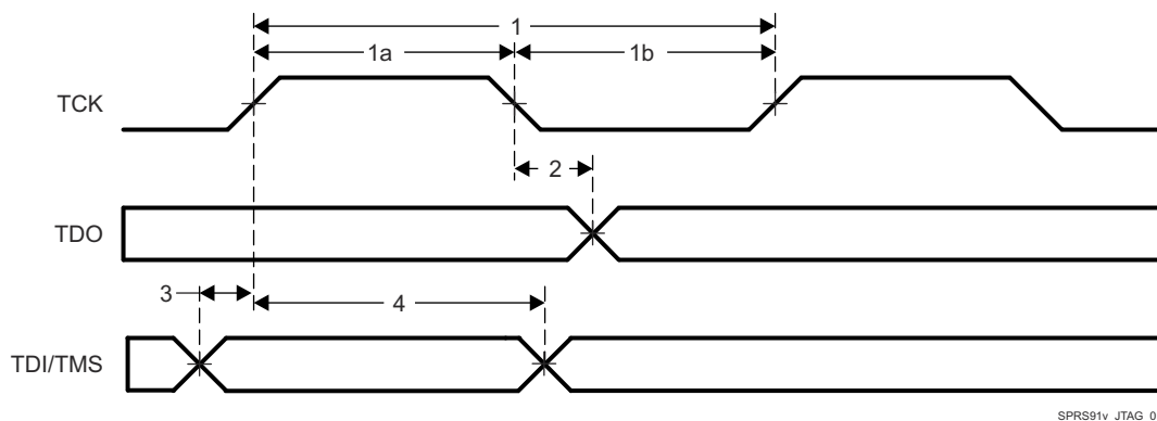
図 6-25. JTAG Timing
