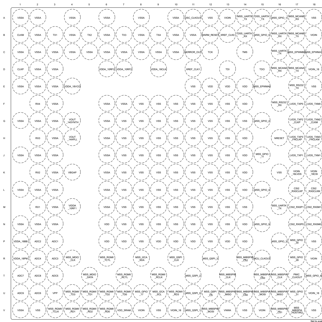
图 5-1. Pin Diagram
