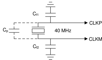
図 6-3. Crystal Implementation
