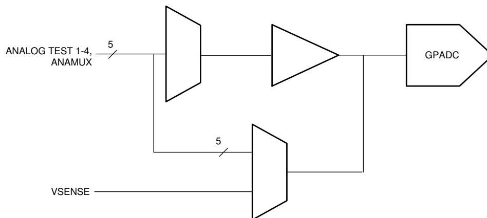
図 8-6. ADC Path
