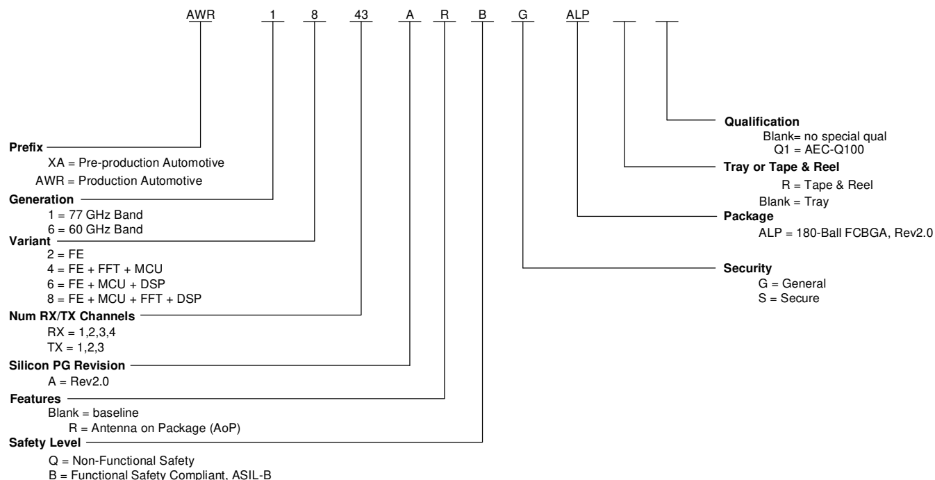
図 10-1. Device Nomenclature
