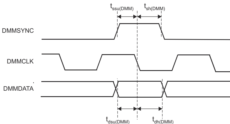
図 6-23. DMMDATA Timing
