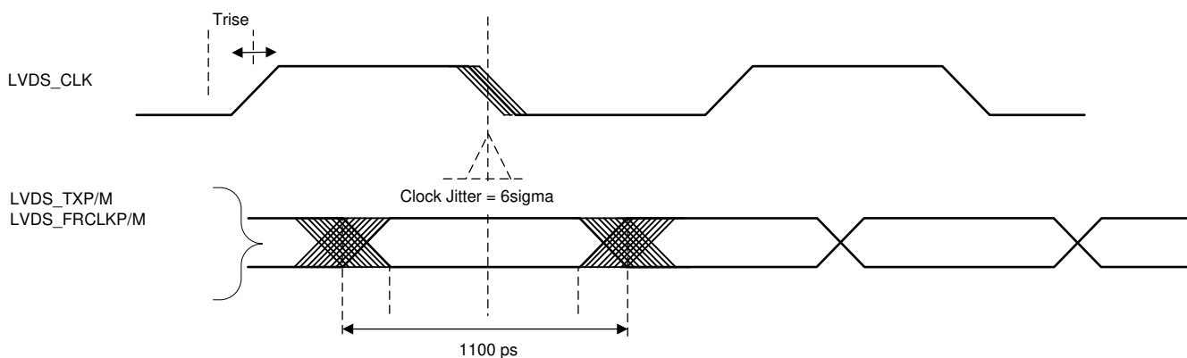
❏ 6-16. Timing Parameters
