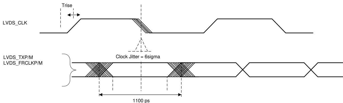
図 8-13. Timing Parameters
