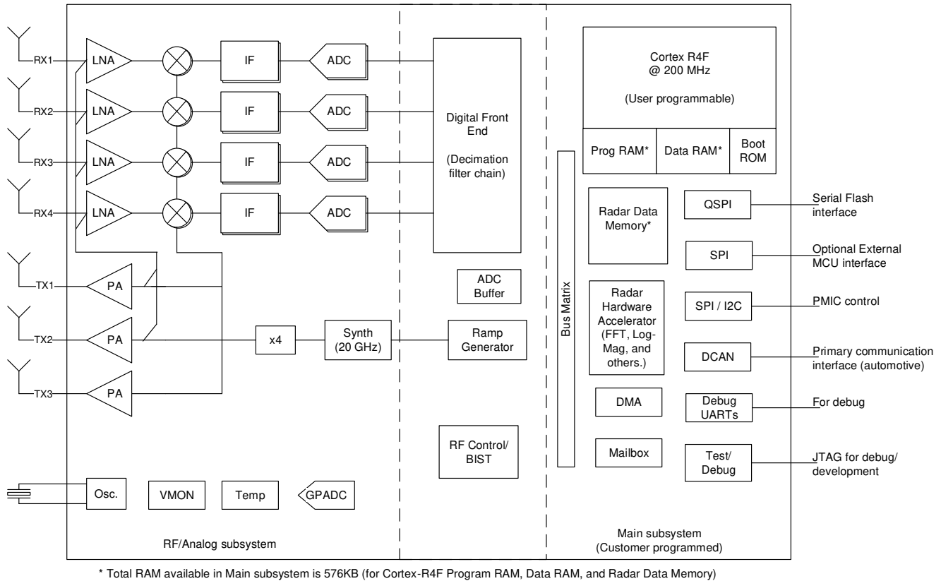
図 4-1. 機能ブロック図
