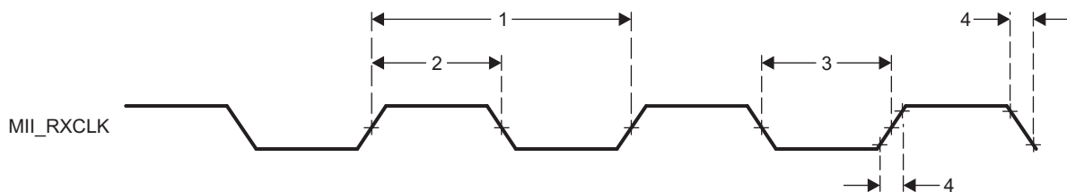
図 7-94. PRU-ICSS MII_RXCLK Timing
