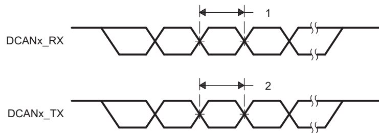
図 7-1. DCANx Timings
