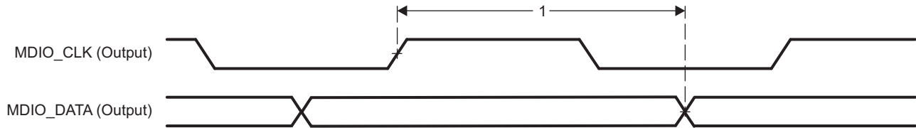
図 7-93. PRU-ICSS MDIO_DATA Timing – Output Mode
