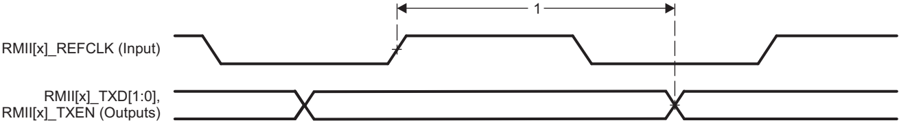
図 7-12. RMII[x]_TXD[1:0], RMII[x]_TXEN Timing - RMII Mode
