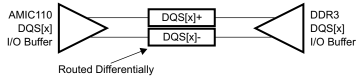
7-62. DQS[x] Topology
