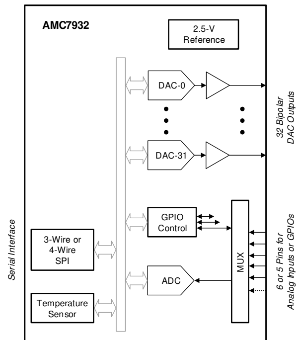
概略回路図
