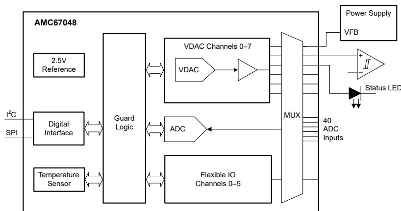
概略回路図
