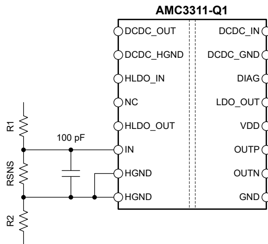
图 8-2. Input Filter
