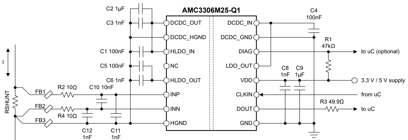
7-4. Decoupling the AMC3306M25-Q1
