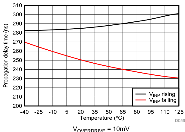
図 5-49. Cmp2 の伝搬遅延と温度との関係
