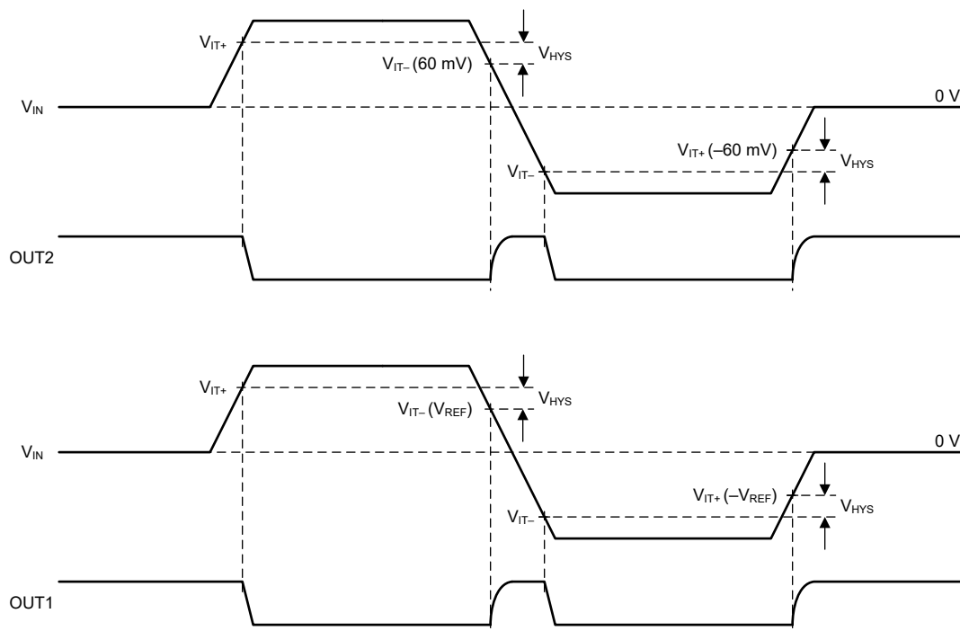
図 6-1. スwitchング スレッショルドとヒステリシス
