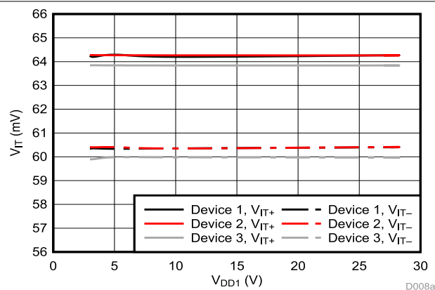
図 5-6. Cmp2 のトリップ スレッシュホールドと電源電圧との関係
