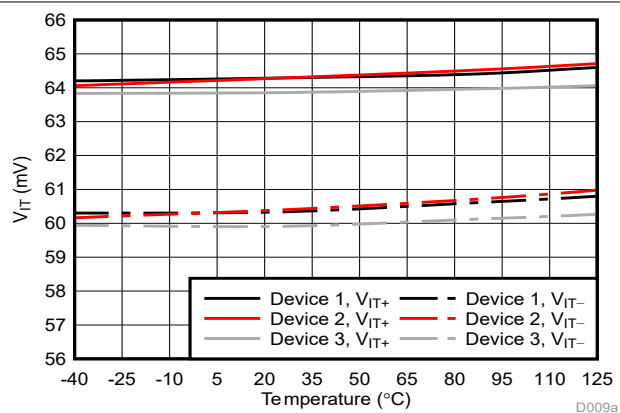
図 5-7. Cmp2 のトリップ スレッシュホールドと温度との関係
