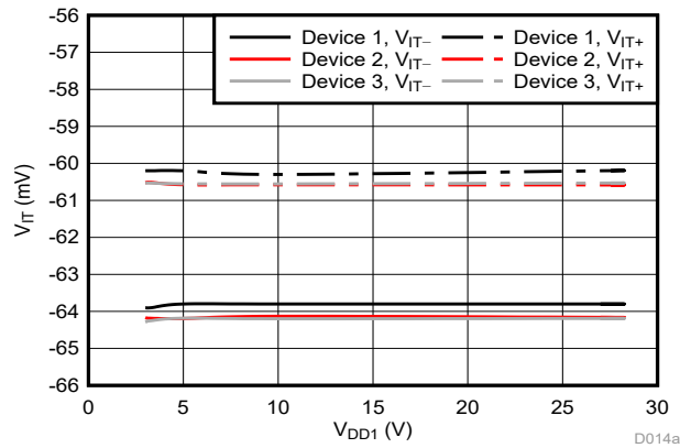
図 5-12. Cmp3 のトリップスレッシュホールドと電源電圧との関係
