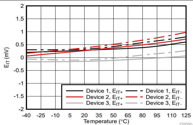
図 5-7. Cmp2 のトリップ スレッシュホールドと温度との関係
