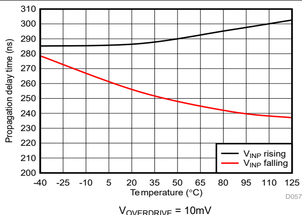
図 5-53. Cmp0 の伝搬遅延と温度との関係
