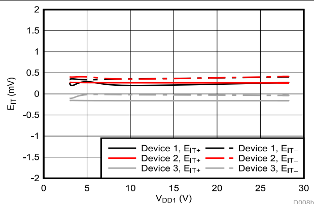
図 5-6. Cmp2 のトリップ スレッシュホールドと電源電圧との関係
