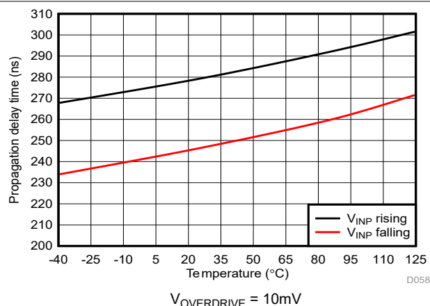
図 5-55. Cmp1 の伝搬遅延と温度との関係
