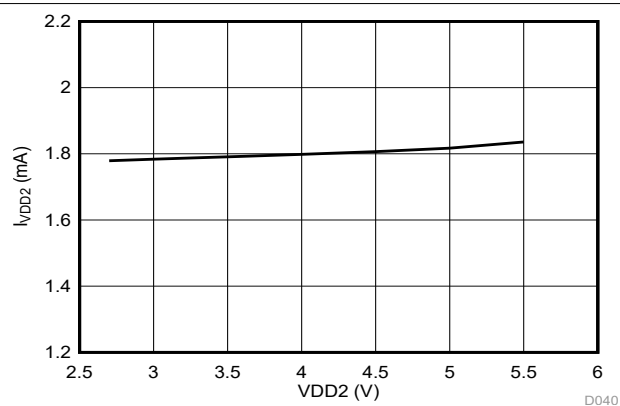
図 5-44. ハイサイド電源電流と電源電圧との関係
